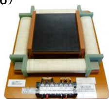
エプスタイン試験器
