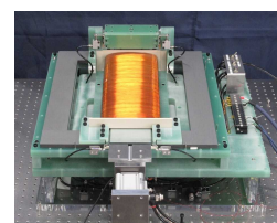
磁歪試験器
