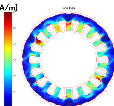
鉄損分布
