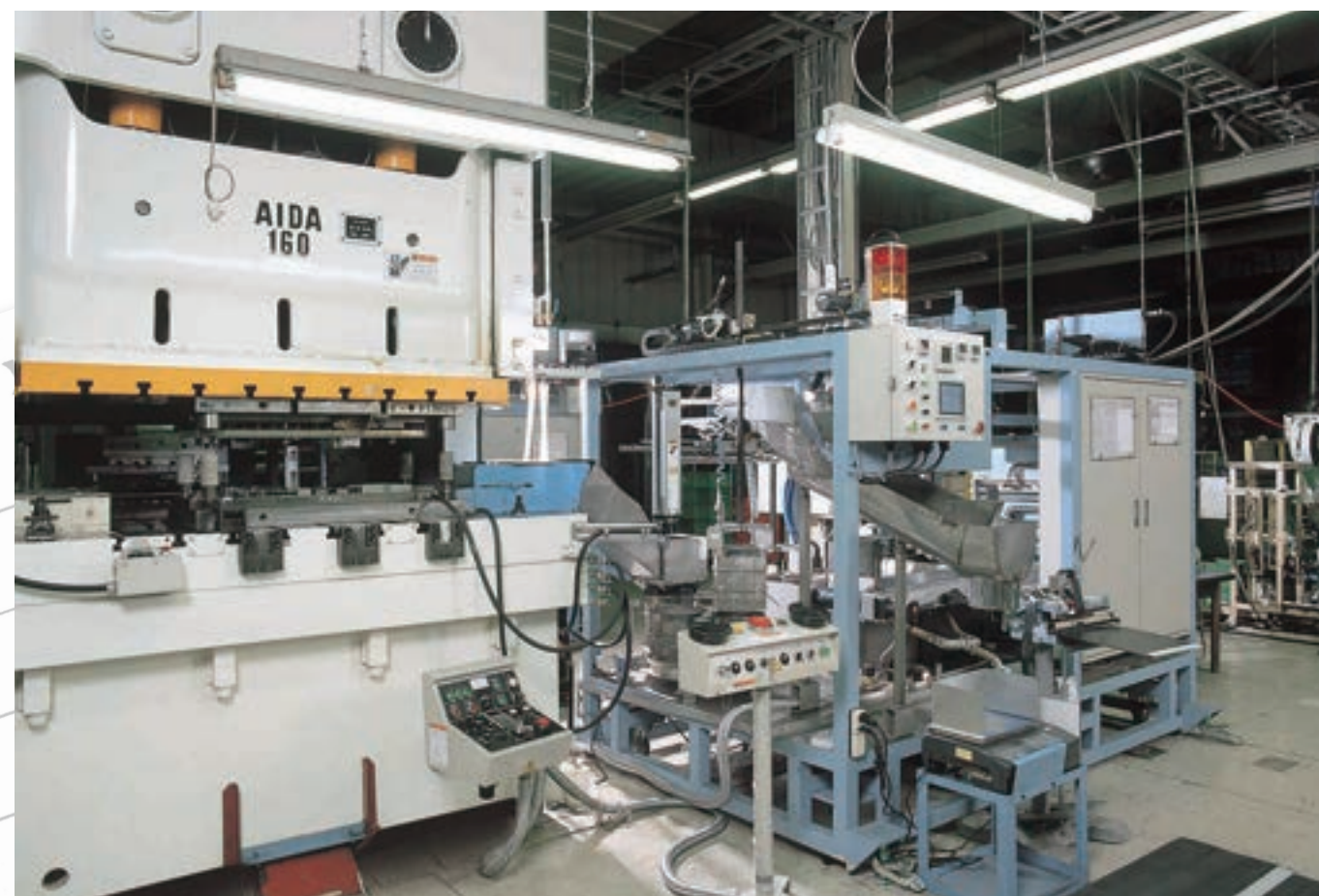
プレス成形洗浄自動化ライン
