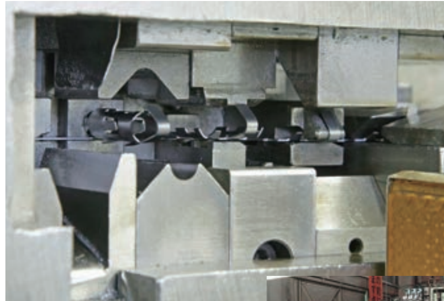
フォーミングマシン
