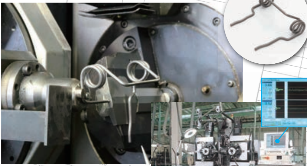
NCスプリングフォーマー
