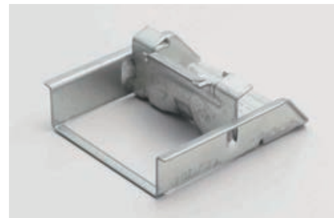
■外装建材固定金具 外装建材の取付金具です。金具側面を有効利用し、金具強度、外装材の保持力を向上させています。
