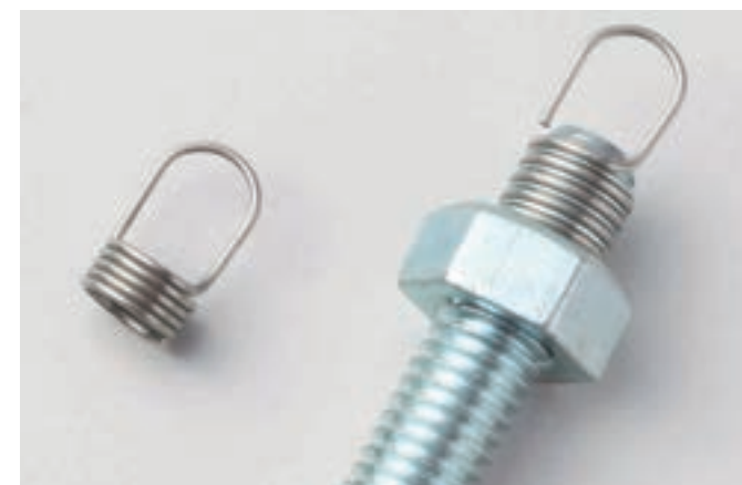
■脱落防止具 ばねがボルトねじ谷部に入り込み塞ぐ事で振動によるナットの脱落を防ぎ、安全性の向上や作業性の省力化を可能にしました。
