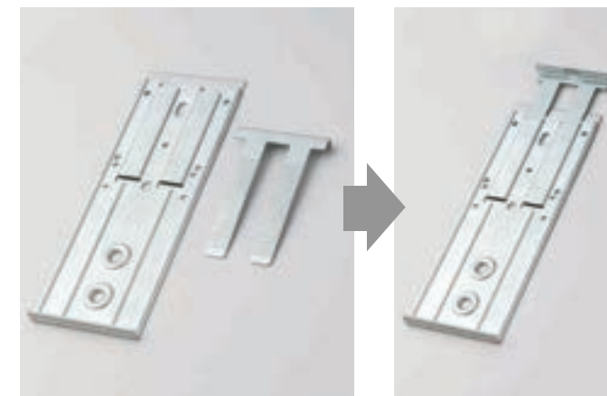
■外装建材固定金具 外装建材の取付金具です。複数の固定部材を着脱可能に組合せ、建材の取付及び取り外しを容易にし、取付強度を向上させています。
