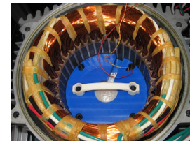
2次元単板磁気試験器
